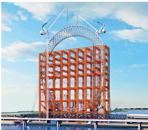
△ 超大直径斜交网格无轴式摩天轮关键施工技术
